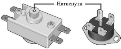
Малюнок 2. Можливі схеми розташування штока (кнопки) термовимикача. Термовимикач знаходиться під нижньою захисною кришкою.
