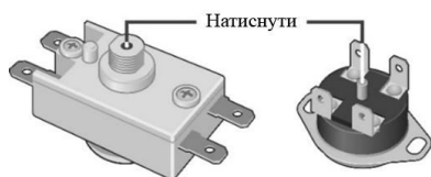
Малюнок 2. Можливі схеми розташування штока (кнопки) термовимикача. Термовимикач знаходиться під нижньою захисною кришкою (панеллю керування)
