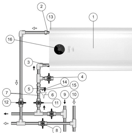
Малюнок 1: 1 – ЕВН, 2 – патрубок гарячої води, 3 – патрубок холодної води, 4 – зливний вентиль, 5 – запобіжний клапан, 6 – дренаж у каналізацію, 7 – підведення, 8 – перекрити вентиль при експлуатації ЕВН, 9 – магістраль холодної води, 10 – магістраль гарячої води, 11 – запірний вентиль холодної води, 12 – запірний вентиль гарячої води, 13 – захисна кришка, 14 – дренажний вихід запобіжного клапана, 15 – ручка для відкривання запобіжного клапана, 16 – ручка керування.
