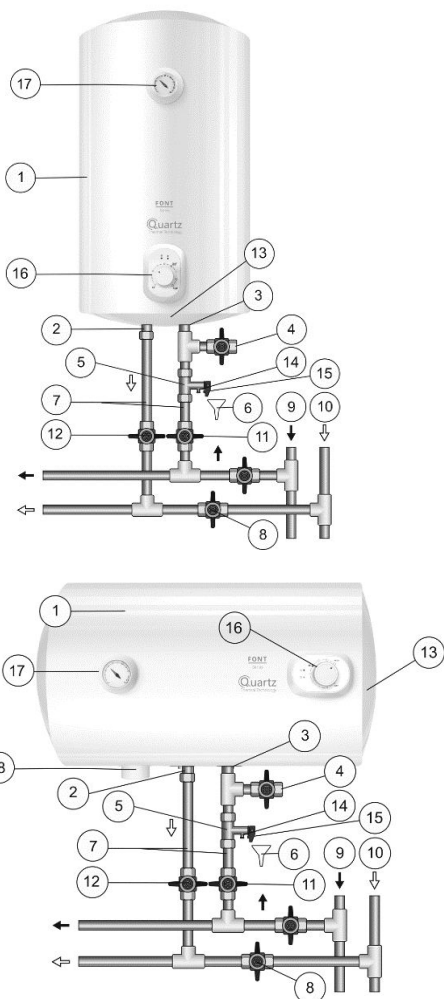
Малюнок 1. Схема підключення ЕВН до водопроводу
