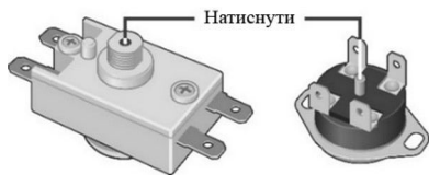
Малюнок 4. Можливі схеми розташування штока (кнопки) термовимикача. Термовимикач знаходиться під нижньою захисною кришкою (панеллю керування)
