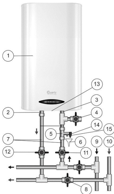
Малюнок 1. Схема підключення ЕВН до водопроводу в вертикальному положенні
