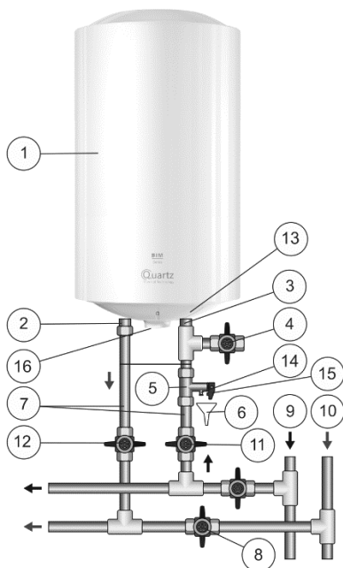
Малюнок 1. Схема підключення ЕВН до водопроводу
