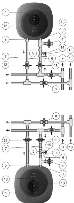
Малюнок 1. Схема підключення ЄВН до водопроводу для моделей Betlis U (патрубки вгору) та Betlis O (патрубки вниз)
